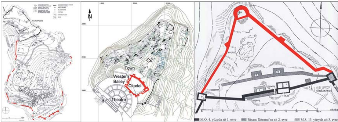
Şekil 3. Pergamon ve Miletos (Tiyatro Tepesi) ve Priene akropolis kent duvarları (Rheidt, 2002, Şekil 2; Niewöhner, 2017, 262 ve Rumscheid, 2000, 220 üzerinden düzenlenmiştir.)
